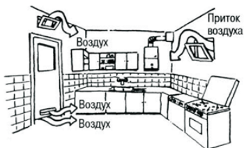
Рис. 4. Монтаж газового водонагревателя
